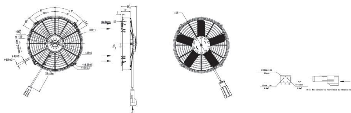
电机外型图 Dimensions:
