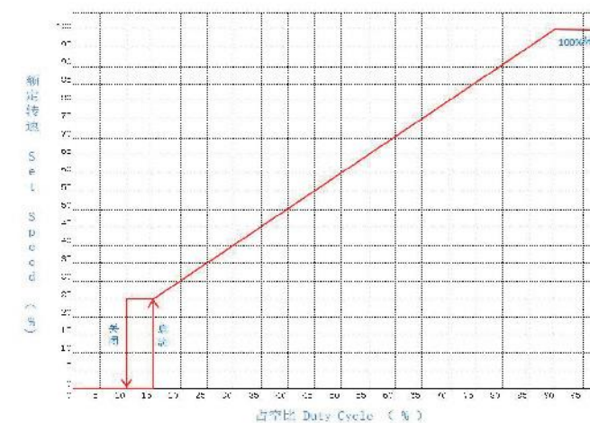
正反转调速 (只支持数字 PWM 信号控制)
