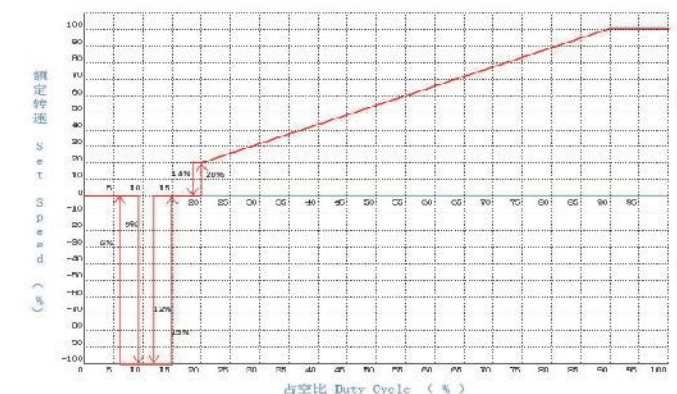
正反转调速 (只支持数字 PWM 信号控制)
