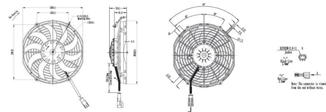
电机外型图 Dimensions:
