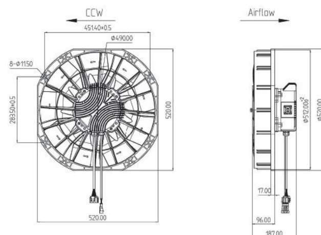
电机外型图 Dimensions:
