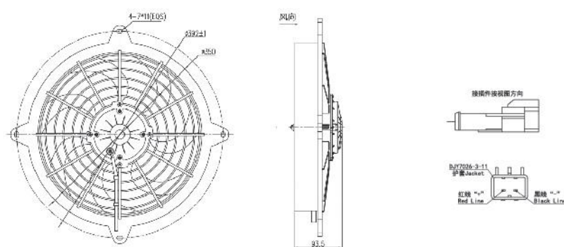
电机外型图 Dimensions:
