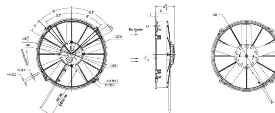
电机外型图 Dimensions:
