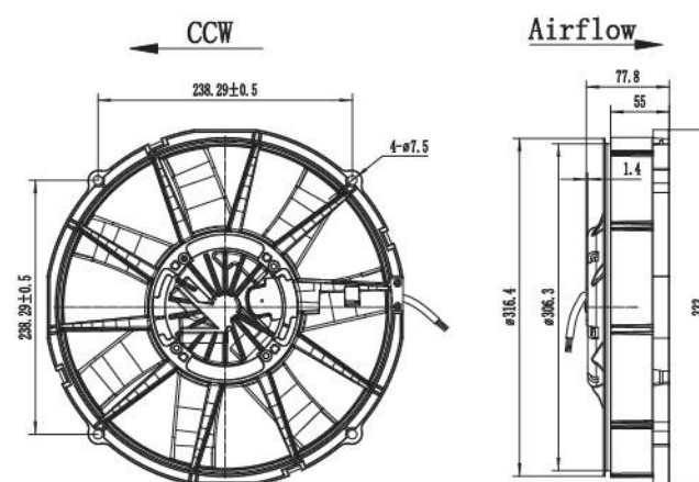
电机外型图 Dimensions:
