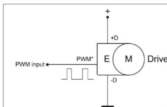
高电平有效数字 PWM 信号调速 (兼容低电平有效数字信号) Digital PWM input/active high(Digital PWM input/active low)
