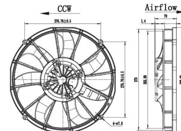
电机外型图 Dimensions:
