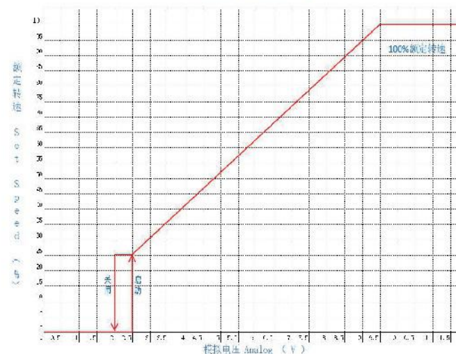
单方向调速 (兼容数字 PWM 信号和模拟电压控制)
