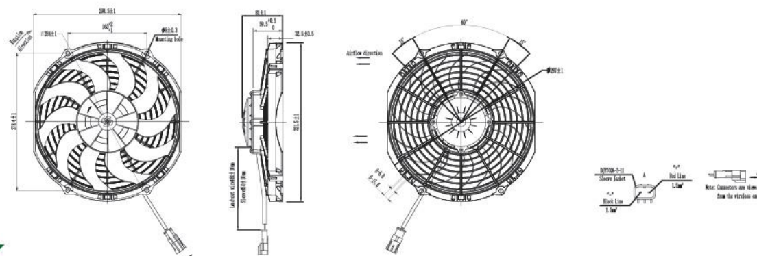
电机外型图 Dimensions:
