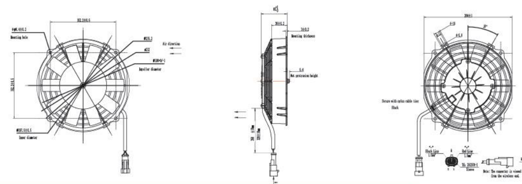
电机外型图 Dimensions:
