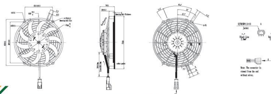
电机外型图 Dimensions:
