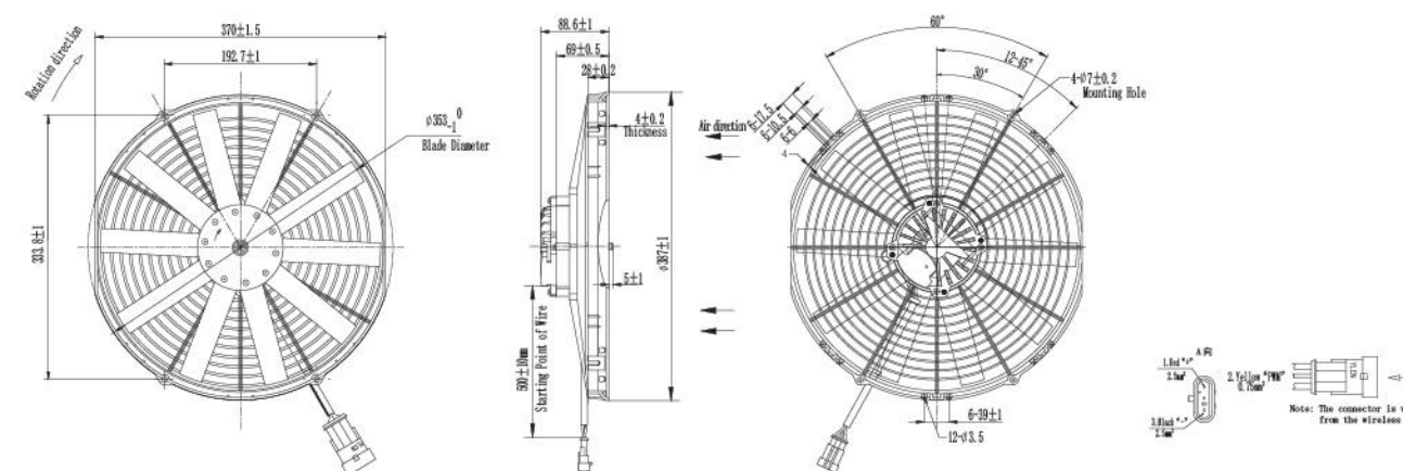
电机外型图 Dimensions:
