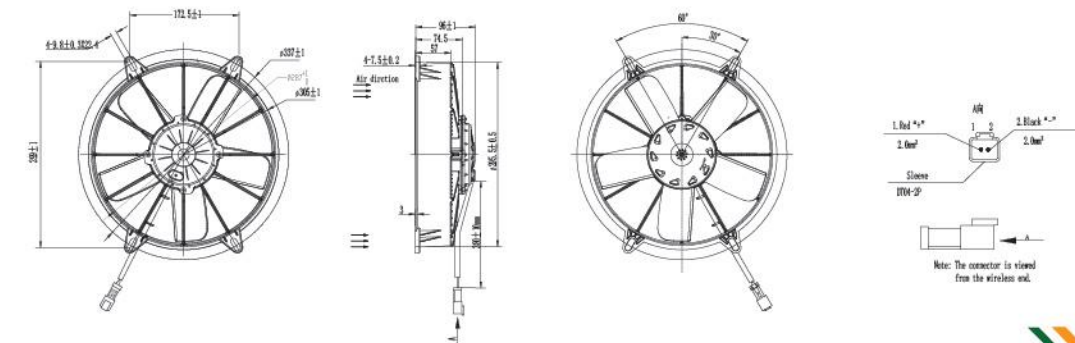
电机外型图 Dimensions:
